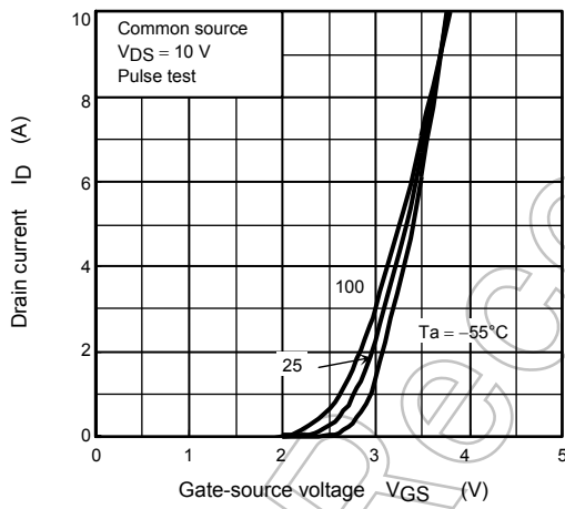
I_D - V_{GS}
