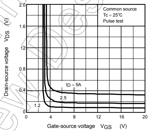
V_{DS} - V_{GS}
