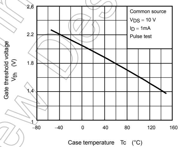
V_{th} - T_c
